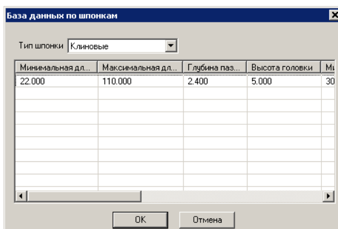
Рис. 3.15 База данных по шпонкам
