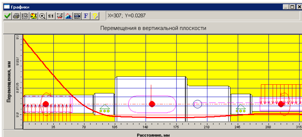
Рис. 3.39 График перемещений в вертикальной плоскости
