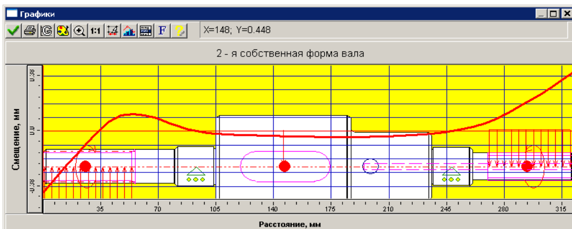
Рис. 3.43 2-я собственная форма изгибных колебаний вала
