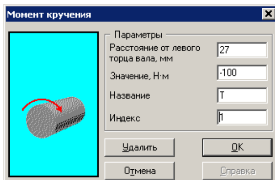
Рис. 3.29 Диалоговое окно ввода и редактирования моментов кручения
