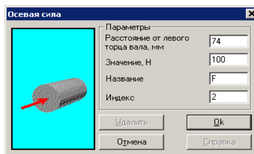
Рис. 3.26 Диалоговое окно ввода и редактирования осевой силы
