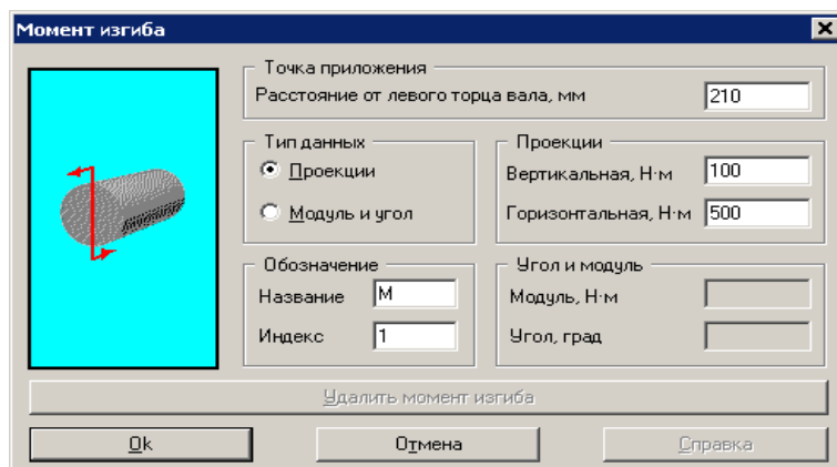
Рис. 3.28 Диалоговое окно ввода и редактирования момента изгиба
