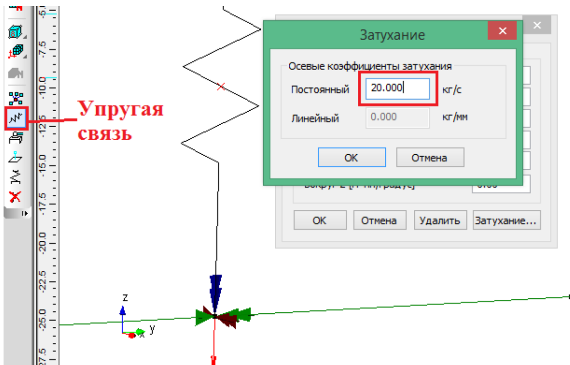
Рисунок 13.19 – Найденное постоянное значение коэффициента затухания
