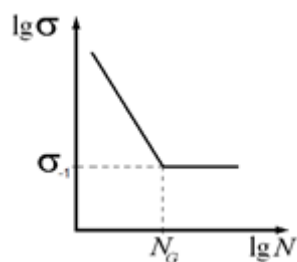
Рисунок 7.14 – Кривая Велера для углеродистой и среднелегированной стали.
