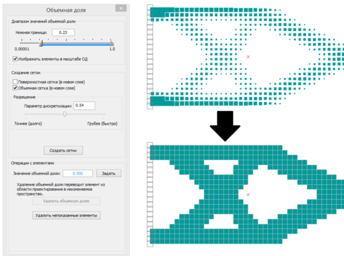
Рисунок 11.6 – Показ распределения объемной доли в конструкции через окно Объемная доля. Сверху – отображение элементов в масштабе объемной доли, снизу – без масштаба объемной доли
