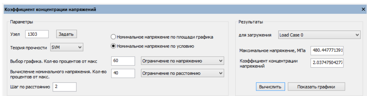
Рисунок 11.21 – Диалоговое окно "Коэффициент концентрации напряжений" с результатами
