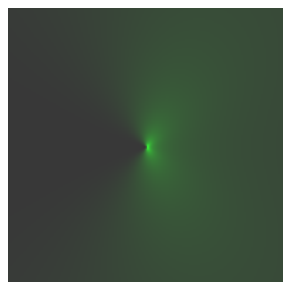
Рисунок 7.3 – Напряжения у фронта трещины
