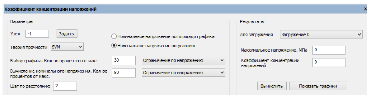
Рисунок 11.13 – Диалоговое окно "Коэффициент концентрации напряжений"
