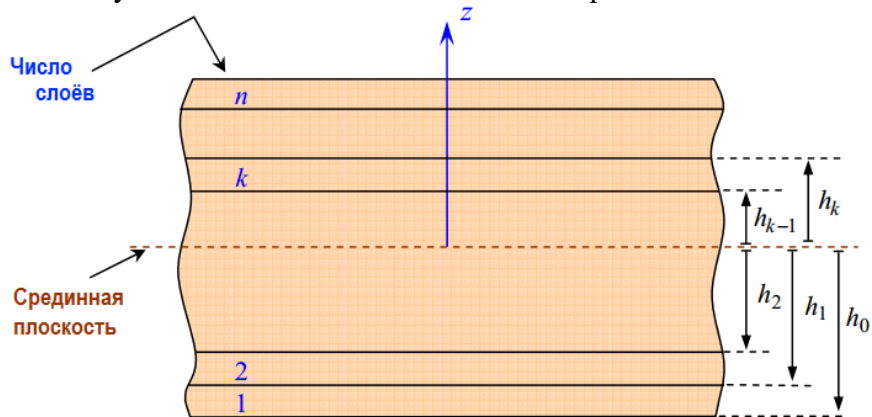
Рисунок 5.13 – Схема расположения слоев ламината в пластине
