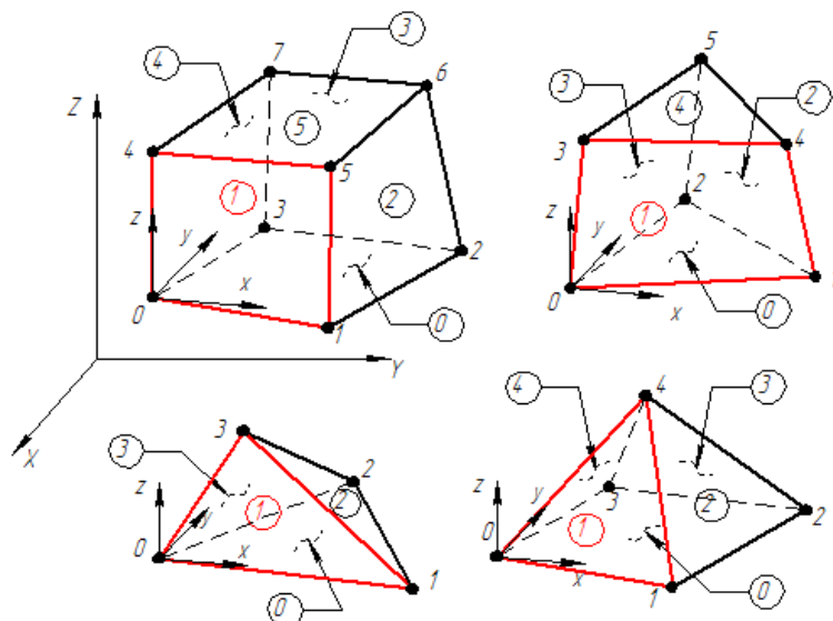
Рисунок 15.6 – Нумерация поверхностей объемных элементов
