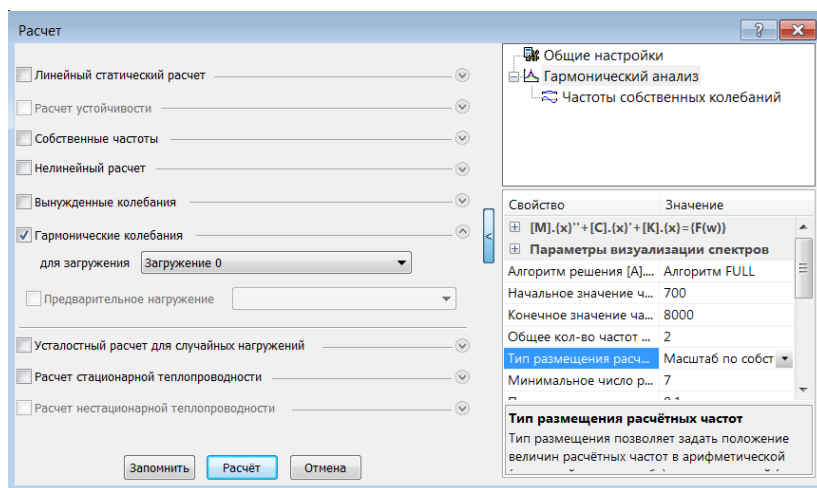
Рисунок 6.9 – а) Диалог запуска на расчет для ГА с отображением настроек расчета б) настройки расчета собственных частот в ГА для случая размещения частот по собственным частотам
