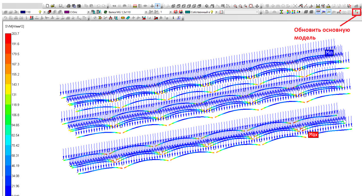
Рисунок 13.10 – Карта результатов напряжений по SVM (Мизесу)
