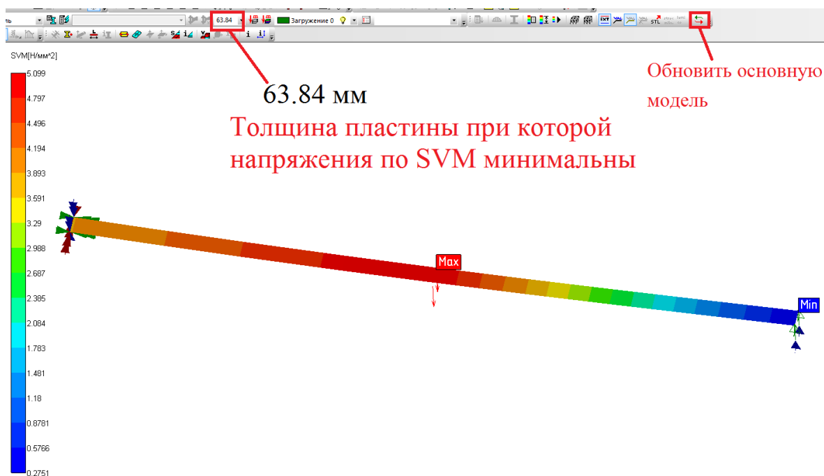
Рисунок 13.5 – Карта результатов напряжений по SVM (Мизесу)
