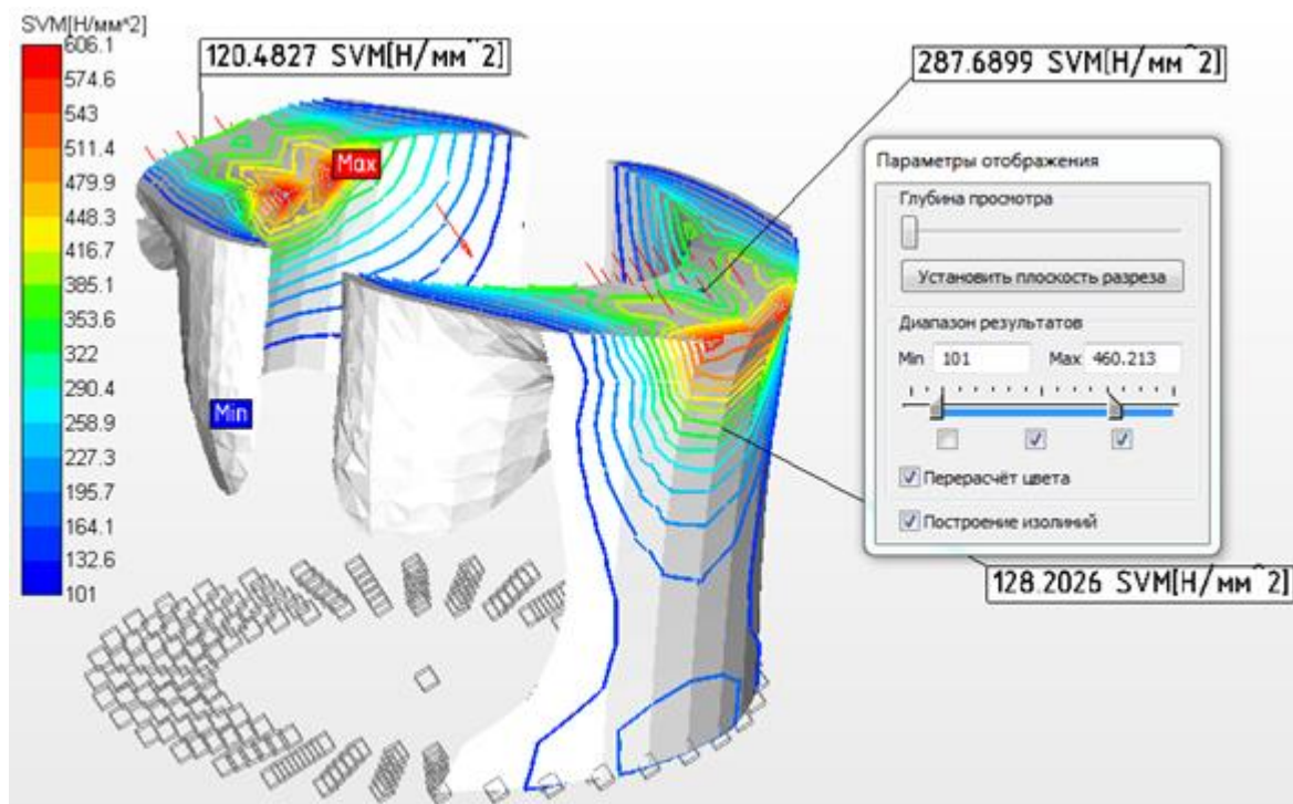
Рисунок 11.5 – Показ части карты напряжений с помощью изолиний на альтернативной карте результатов
