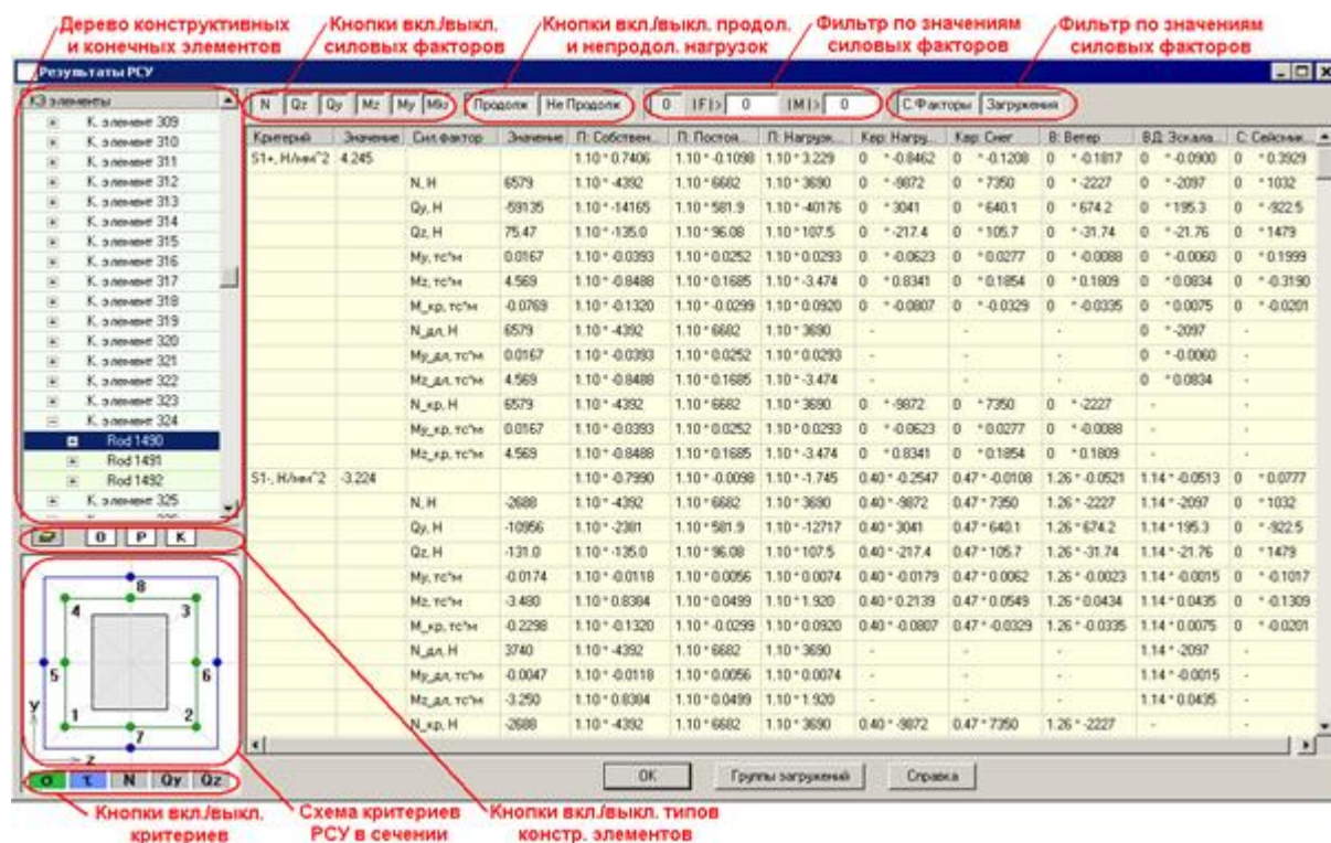
Рисунок 11.8 – Таблица результатов расчета РСУ для стержня
