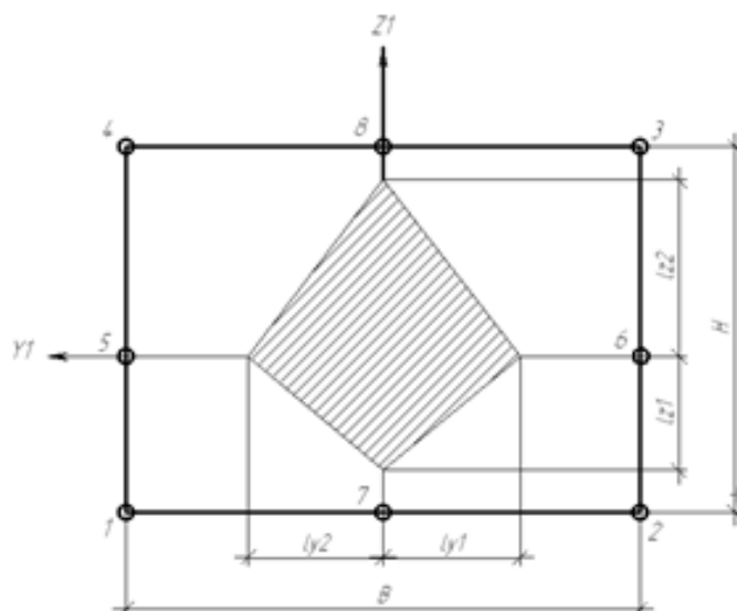
Рисунок 11.9 – Прямоугольник, ограничивающий габариты произвольного сечения.
