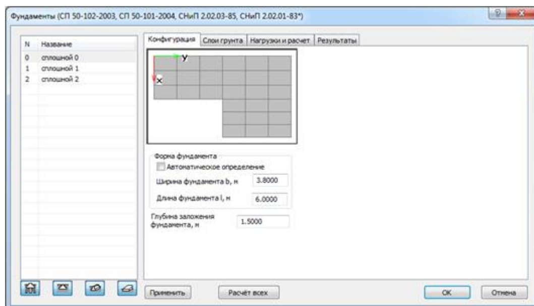
Рисунок 10.3 – Диалоговое окно Фундаменты – конфигурация сплошного фундамента.
