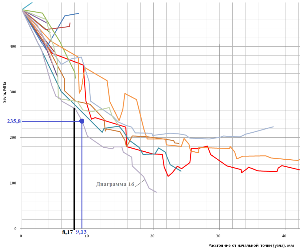
Рисунок 11.20 – Схема нахождения номинального напряжения
