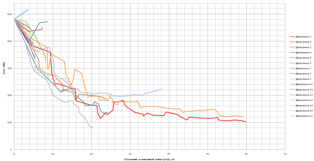
Рисунок 11.18 – Диаграммы, полученные в примере
