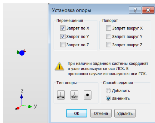
Рисунок 6.1 – Задание закрепления в узлах перед заданием кинематической нагрузки, выбранный узел обозначен большим синим шариком, красная и зеленая стрелки в узел показывают уже заданное закрепления в направлениях X и Y
