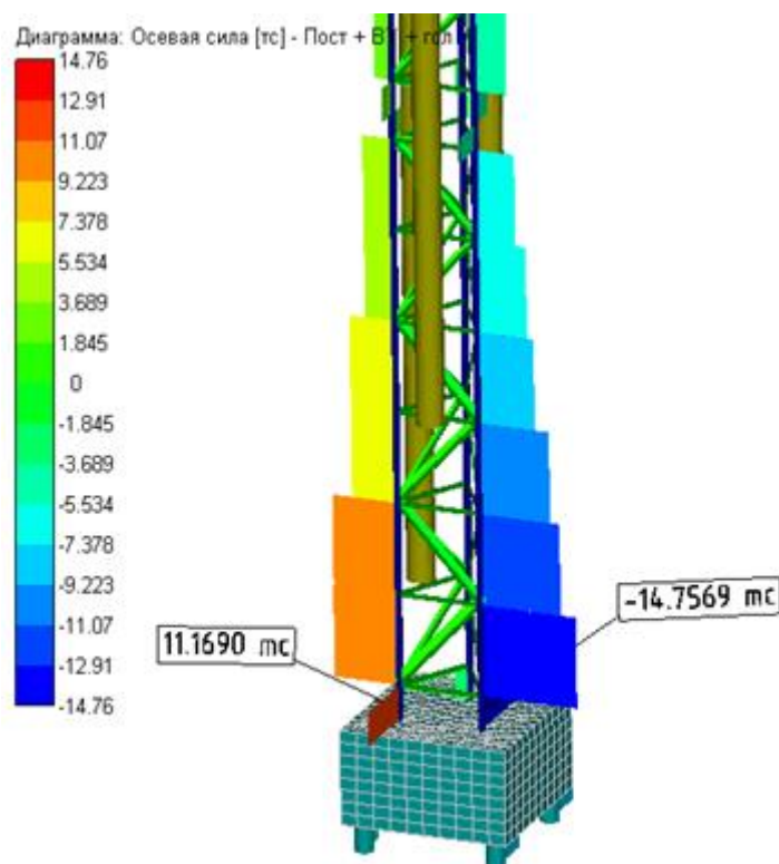
Рисунок 11.1 – Показ эпюр силовых факторов (осевой силы) на стержнях
