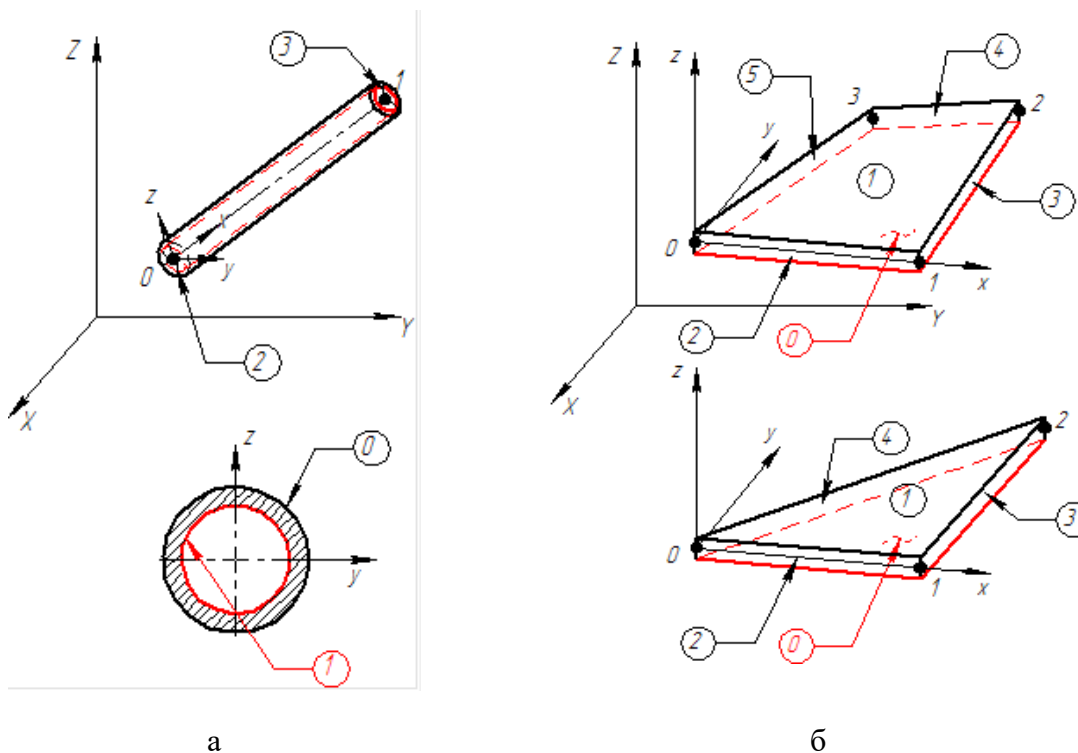
Рисунок 15.5 – Нумерация поверхностей а – стержневого элемента, б – пластинчатого элемента
