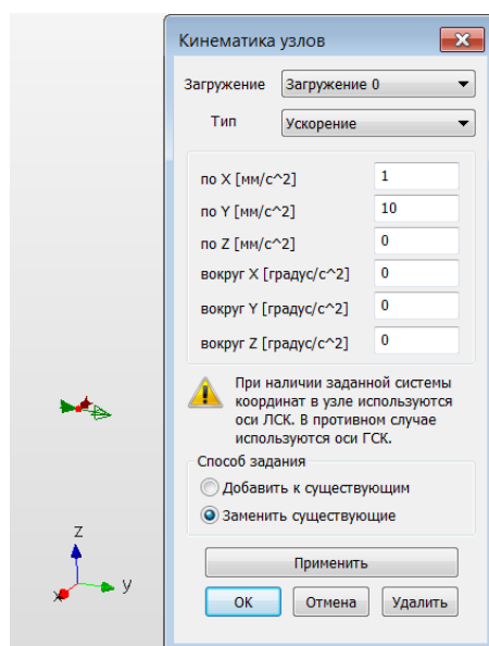
Рисунок 6.2 – Задание кинематической нагрузки, выбранный узел обозначен маленьким красным шариком, итоговое направление кинематической нагрузки показано зеленой стрелкой, выходящей из узла
