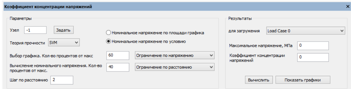
Рисунок 11.17 – Диалоговое окно "Коэффициент концентрации напряжений"
