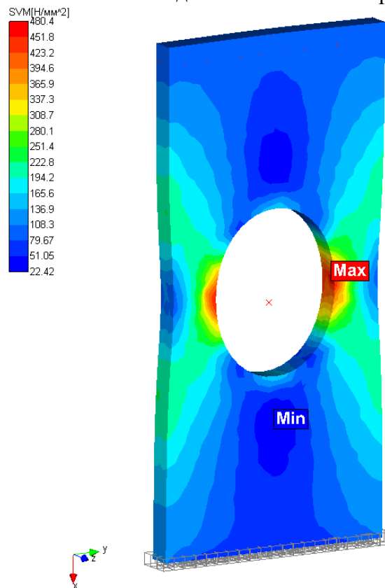
Рисунок 11.16 – Карта результатов эквивалентных напряжений по Мизесу
