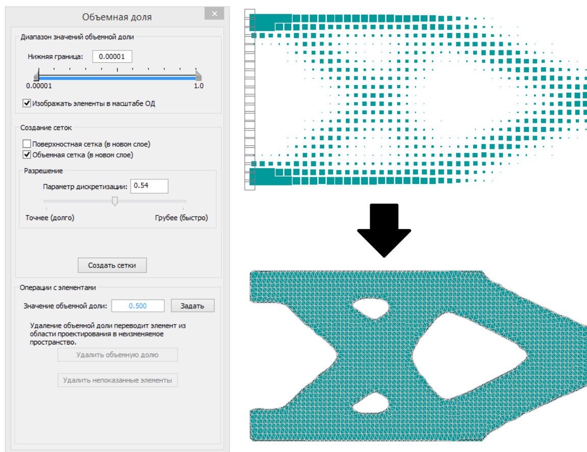
Рисунок 11.7 – Показ результата создания новой сеточной оптимизированной структуры с более мелким шагом по сравнению с исходной
