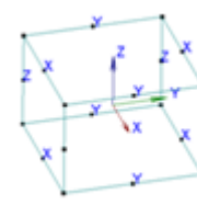
Рисунок 16.1 – Основные типы конечных элементов
