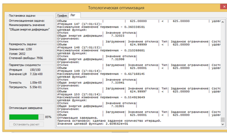
Рисунок 12.11 – Результат оптимизации.
