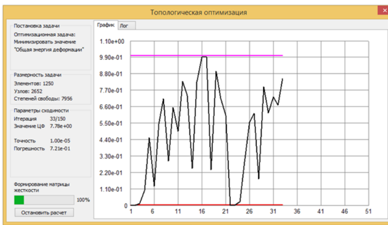
Рисунок 12.10 – Ход оптимизации
