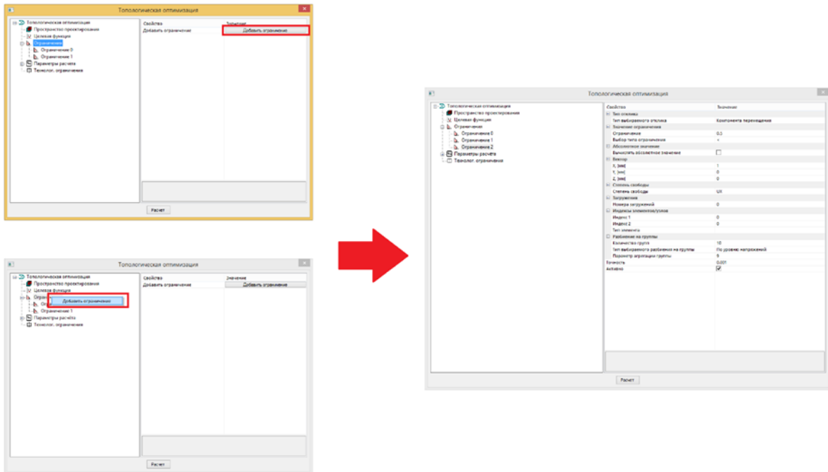
Рисунок 12.5 – Добавление ограничения
