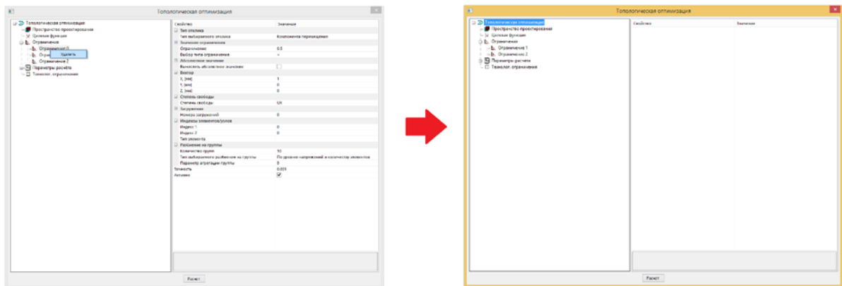
Рисунок 12.6 – Удаление ограничения
