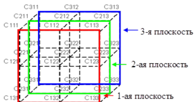
Рисунок 15.2 – Трехмерная матрица
