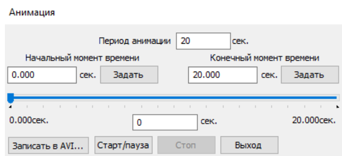
Рисунок 7.28 – Диалог Анимация
