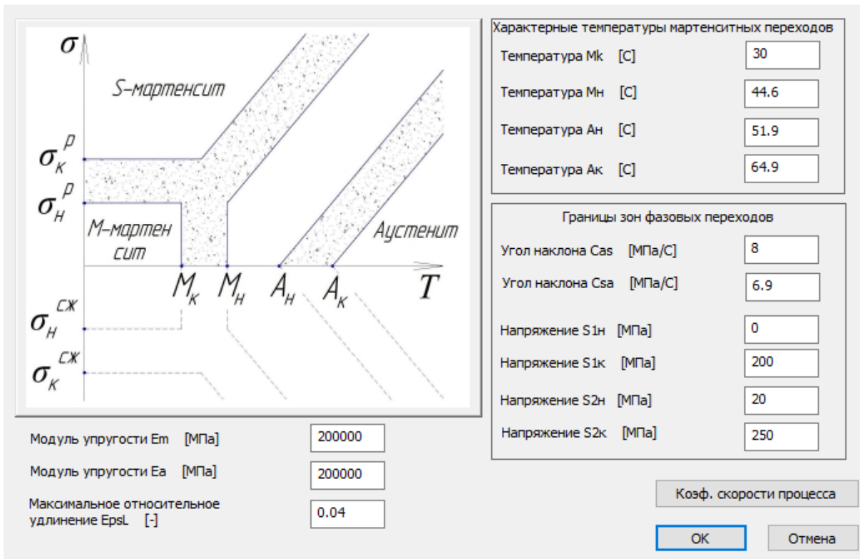
Рисунок 5.5 – Диалог Свойства SMA
