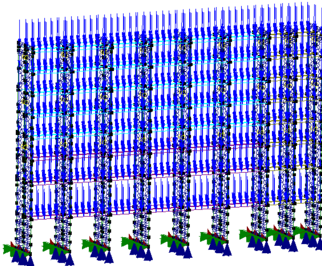
Рисунок 13.6 – Конечно-элементная модель стеллажа
